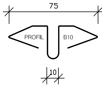
B - PROFIL
