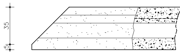
PLATTE MIT GEHRUNGSSCHNITT LINKS + RECHTS
