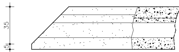
PLATTE MIT GEHRUNGSSCHNITT LINKS
