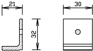
L- holder
