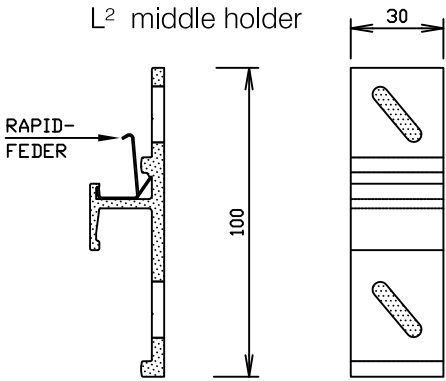
L 2 M-HALTER
