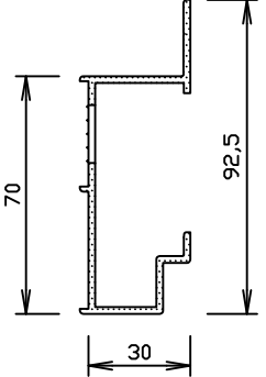
L 2 HF ENDPROFIL
