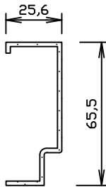
L 2 HF Verbindungsprofil connectong profiles
