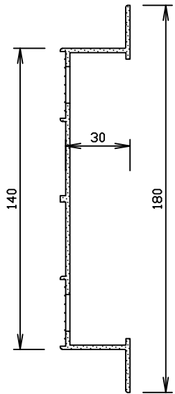
L 2 HF TRAGPROFIL
