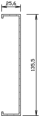
L 2 HF Verbindungsprofil connecting profiles
