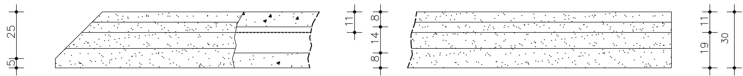
PLAQUE AVEC COUPE D'ONGLET A GAUCHE
