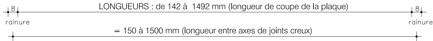
PLAQUE AVEC COUPES D'ONGLETS A DROITE ET A GAUCHE
