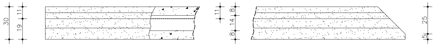
PLAQUE AVEC COUPE D'ONGLET A DROITE
