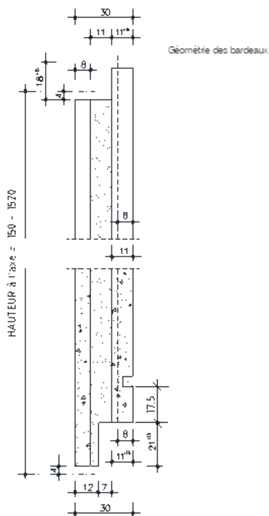
Figure 2 - Géométrie des bardeaux et tolérances dimensionnelles
