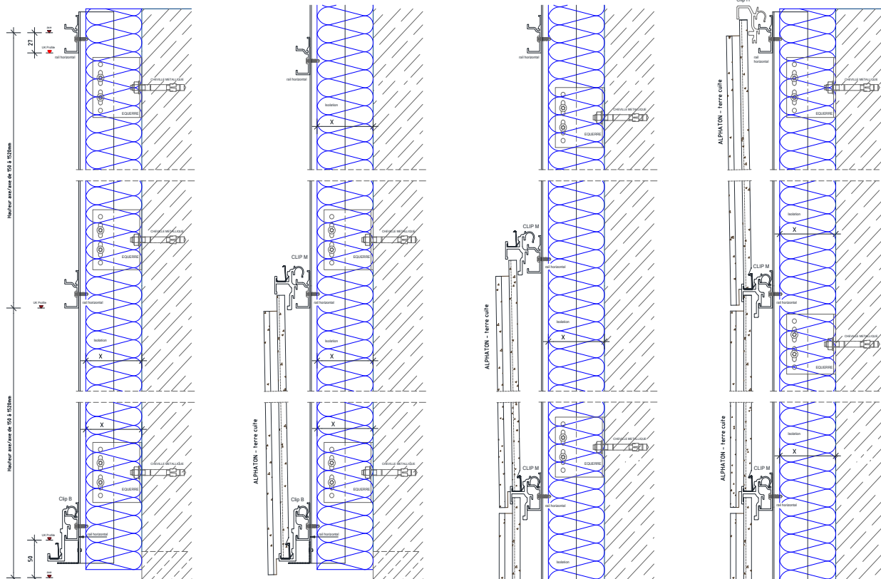
Figure 24 - Montage des bardeaux - méthode 1
