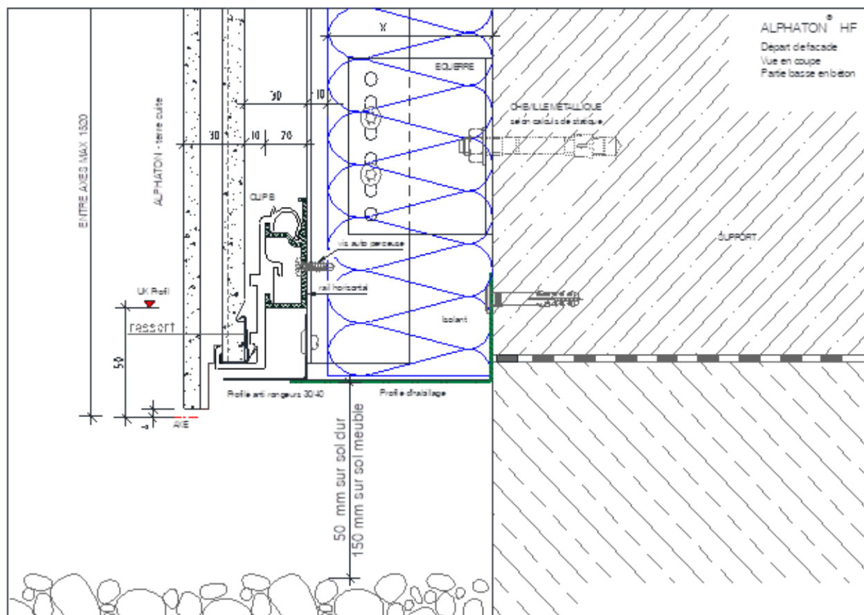
Figure 13 - Départ de façade et socle
