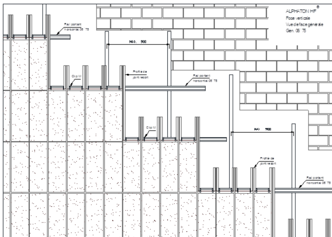
Figure 9 - Vue de face - pose avec rail portant horizontal 06'75
