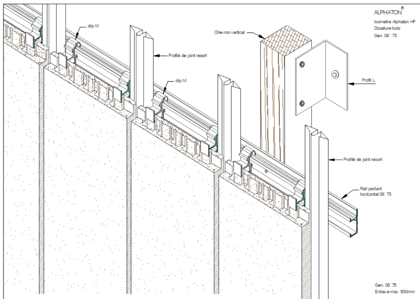
Figure 31 - Vue isométrique
