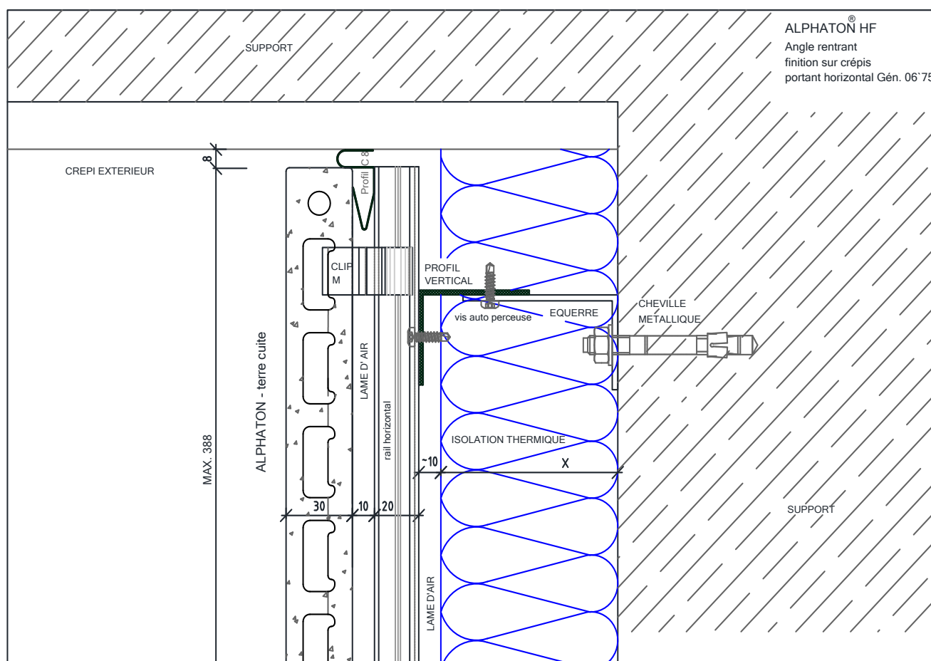
Figure 22- Traitement des angles rentrants - finition sur mur crépis
