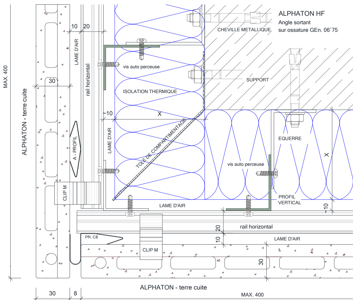
Figure 19 - Traitement des angles sortants - finition avec superposition de plaques
