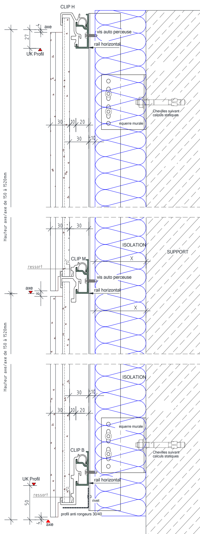
Figure 12 – Coupe verticale avec rail Gén 06'75 ouvert
