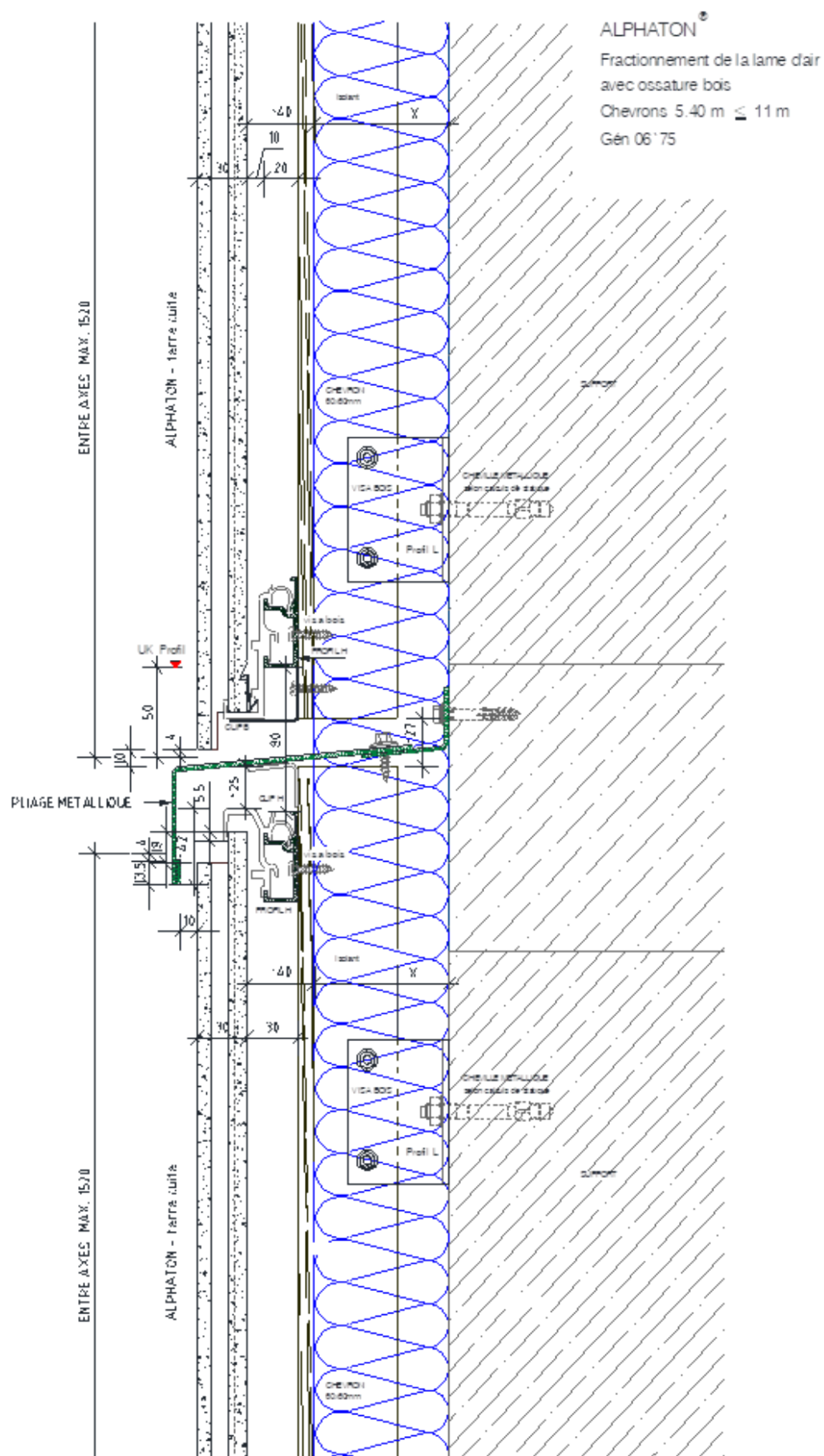
Figure 38 - Fractionnement de la lame d'air
