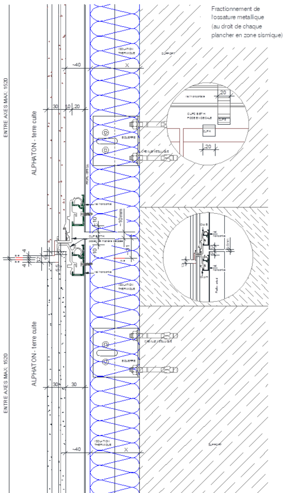
Figure A1 – Fractionnement de l'ossature au droit de chaque plancher sur béton
