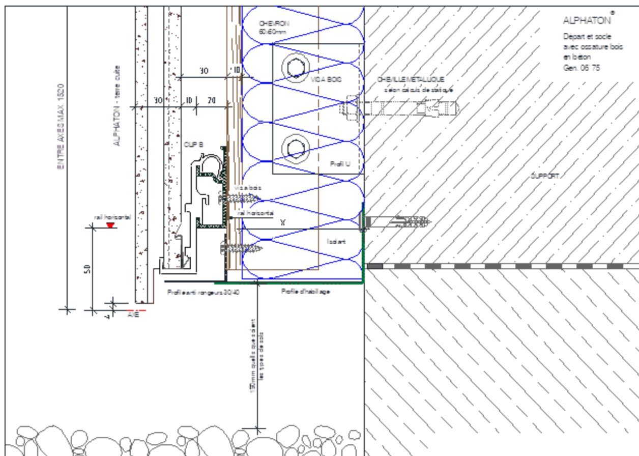
Figure 33 -Départ de façade et socle
