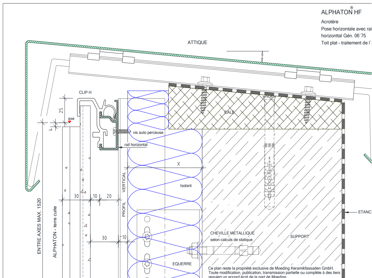
Figure 14 - Acrotère
