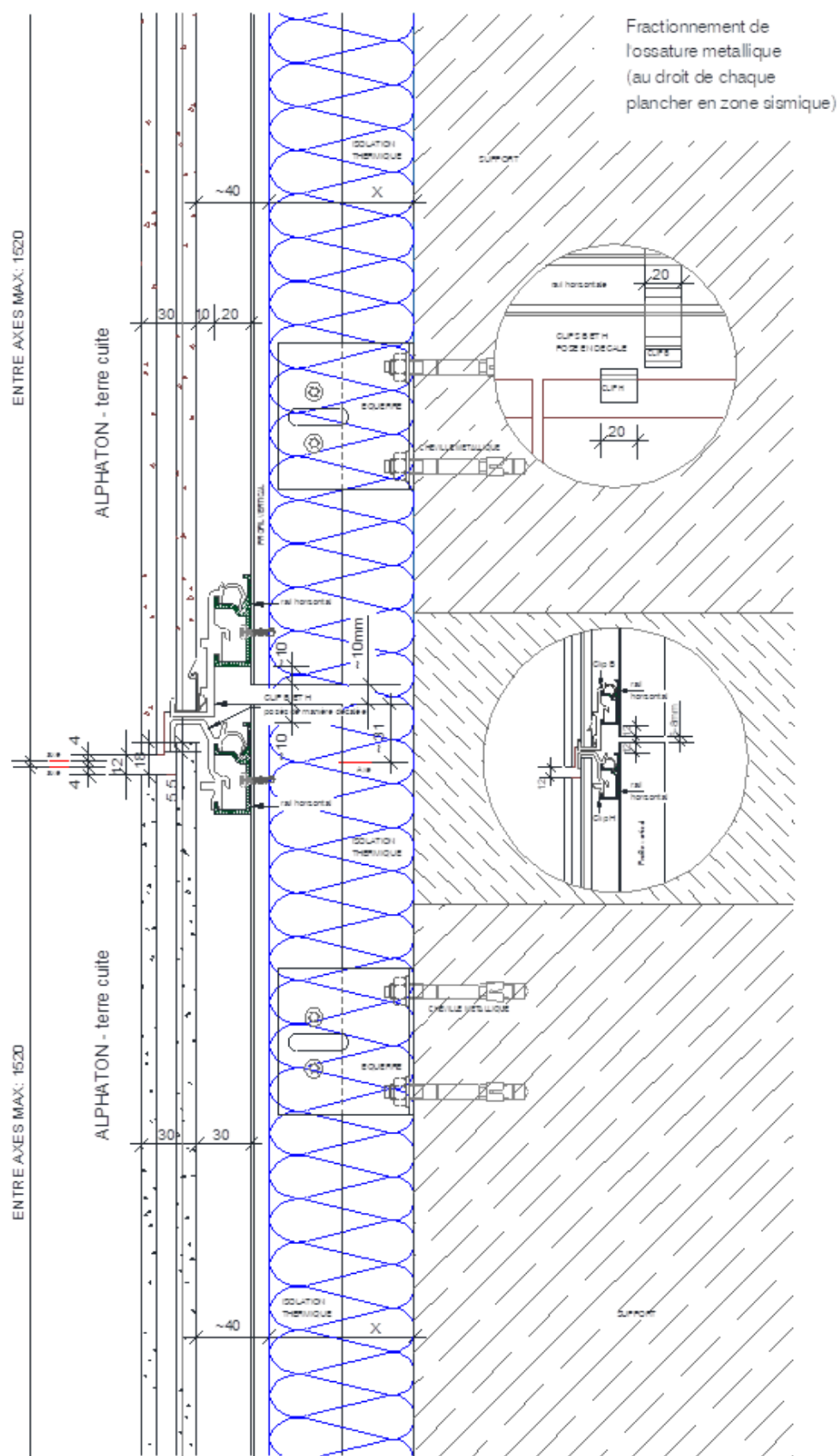
Figure B1 – Fractionnement de l'ossature au droit de chaque plancher sur béton
