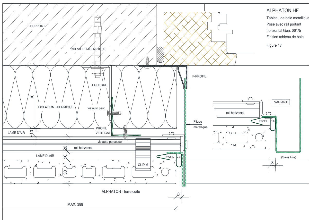
Figure 16 - Tableau de baie métallique
