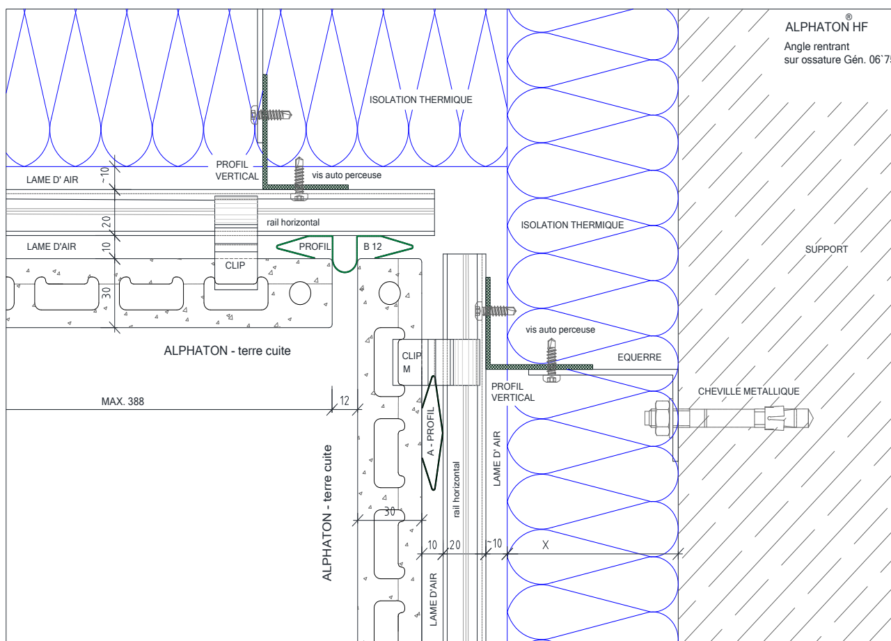
Figure 21- Traitement des angles rentrants
