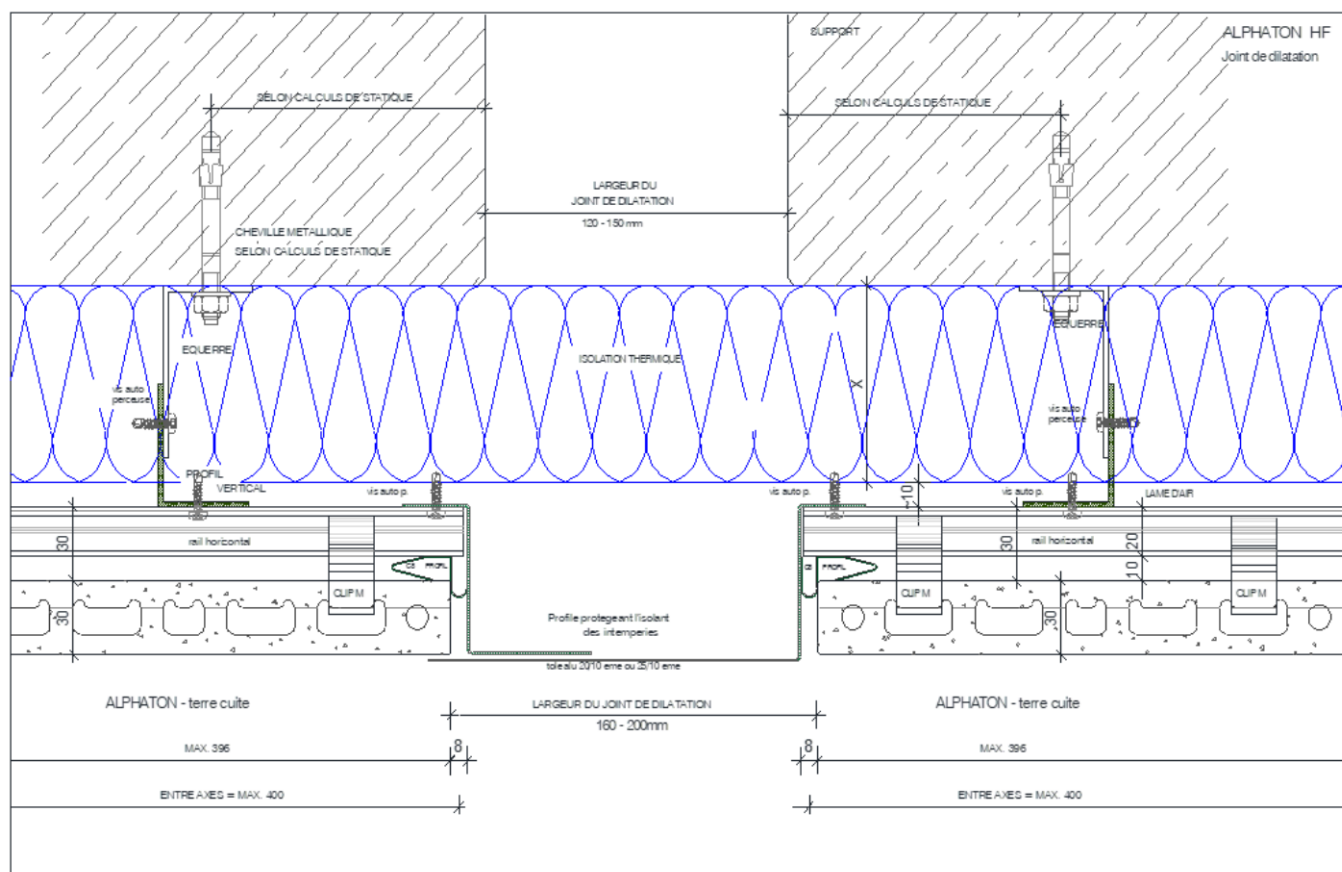
Figure A2 – Détail joint de dilatation de 12 à 15 cm
