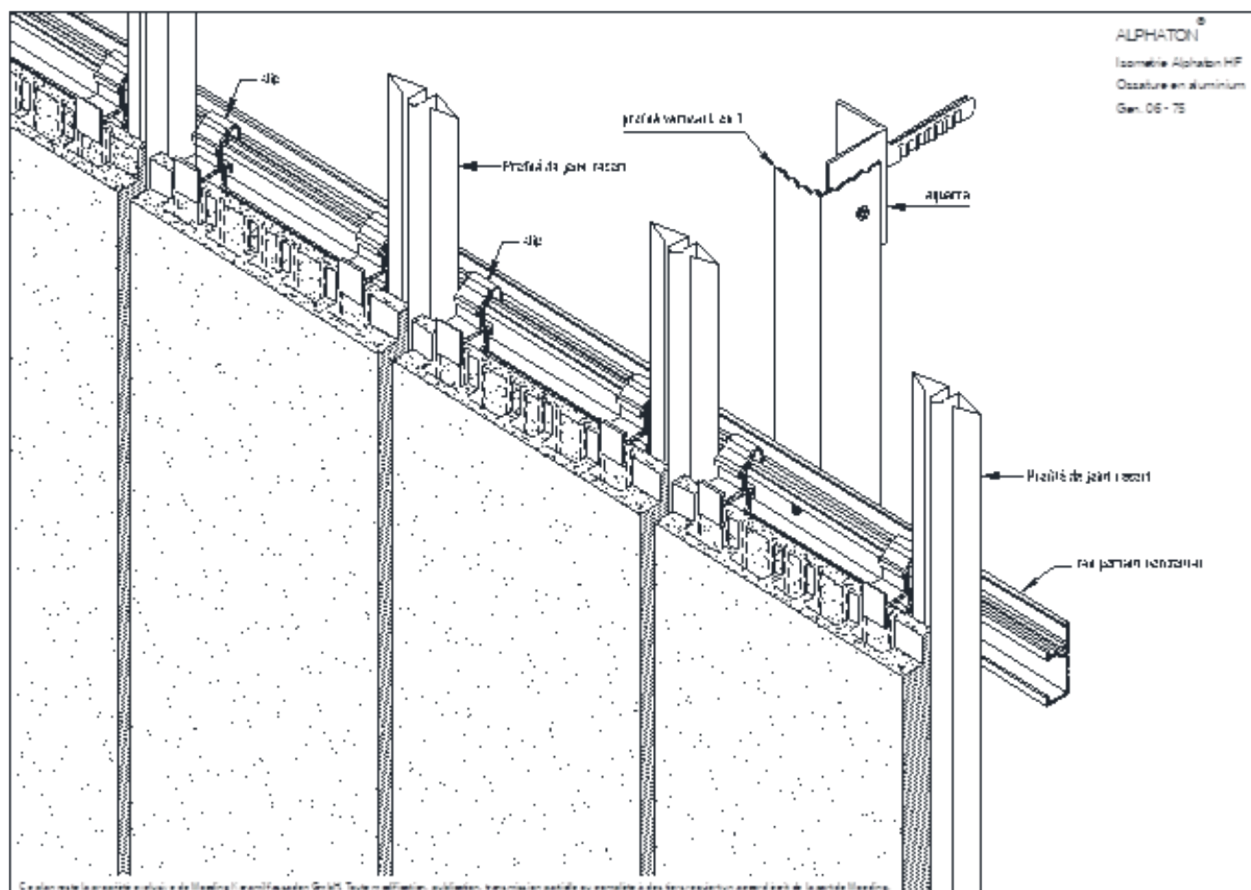
Figure 8 - Schéma de principe ossature métallique - Vue isométrique - pose avec rail portant horizontal 06'75
