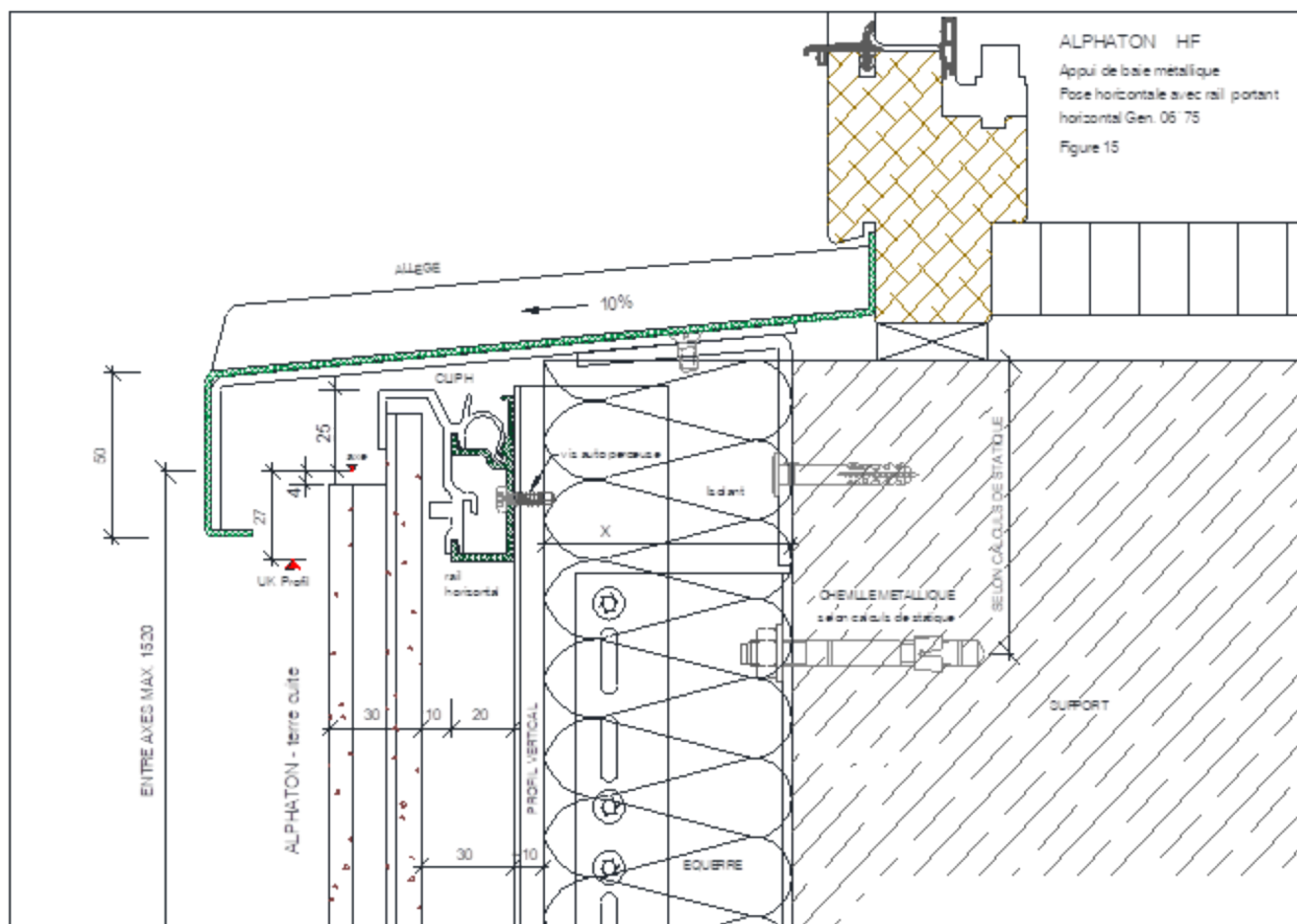
Figure 15 - Appui de baie métallique
