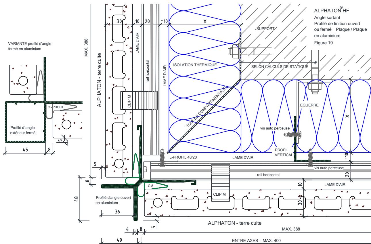
Figure 18 - Traitement des angles sortants - finition avec profilés métalliques d'angle
