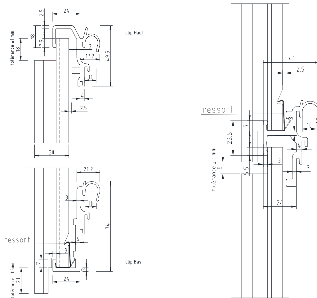
Figure 23 – Prise des bardeaux dans les clips
