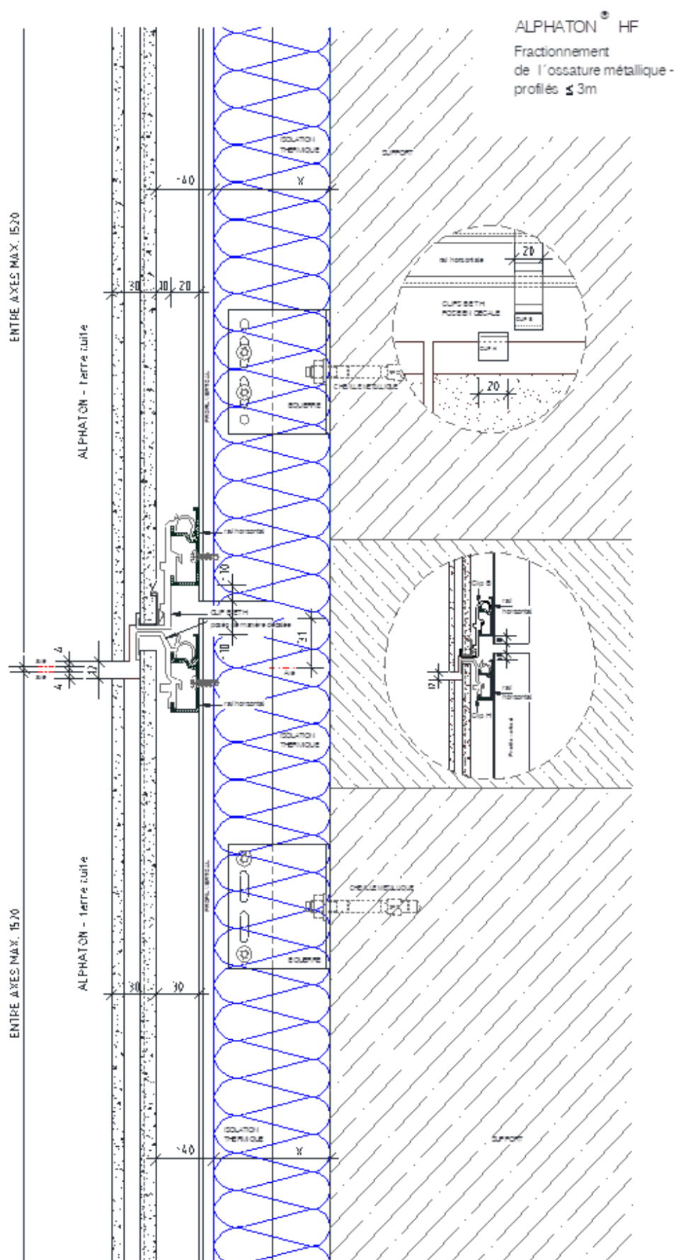
Figure 25 - Fractionnement de l'ossature aluminium librement dilatable – montants de max. 3 m
