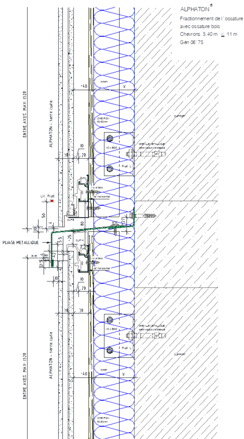
Figure 37 - Fractionnement de l'ossature - Chevrans 5,40m \leq 11m
