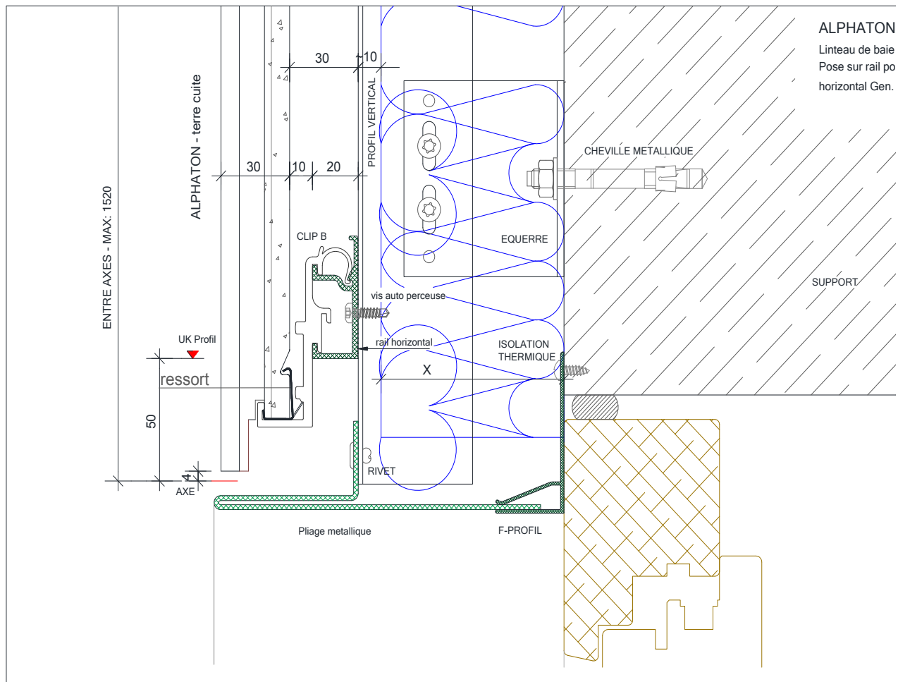
Figure 17 - Linteau de baie métallique
