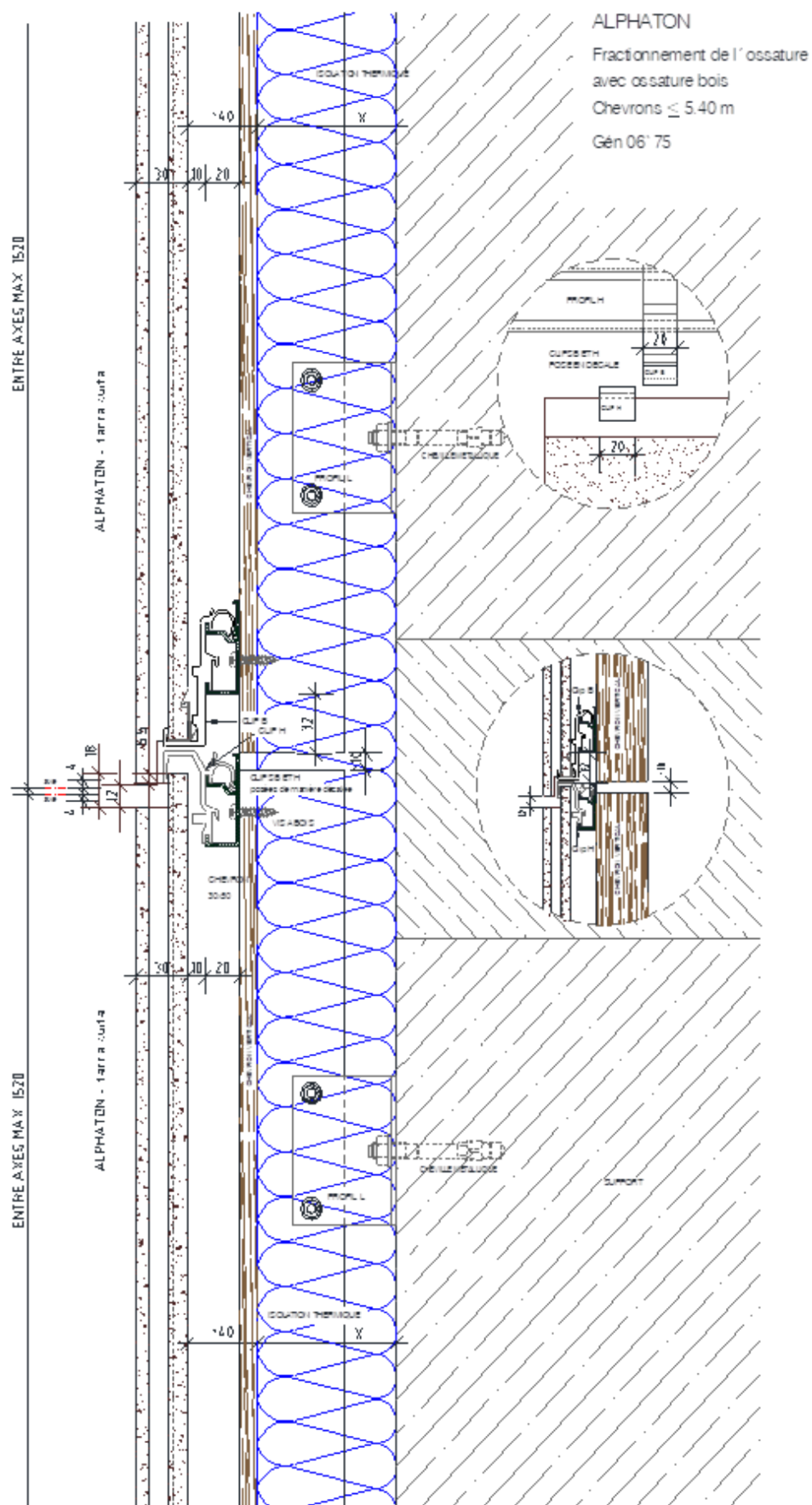
Figure 36 - Fractionnement de l'ossature - Chevrans \leq 5,40 m
