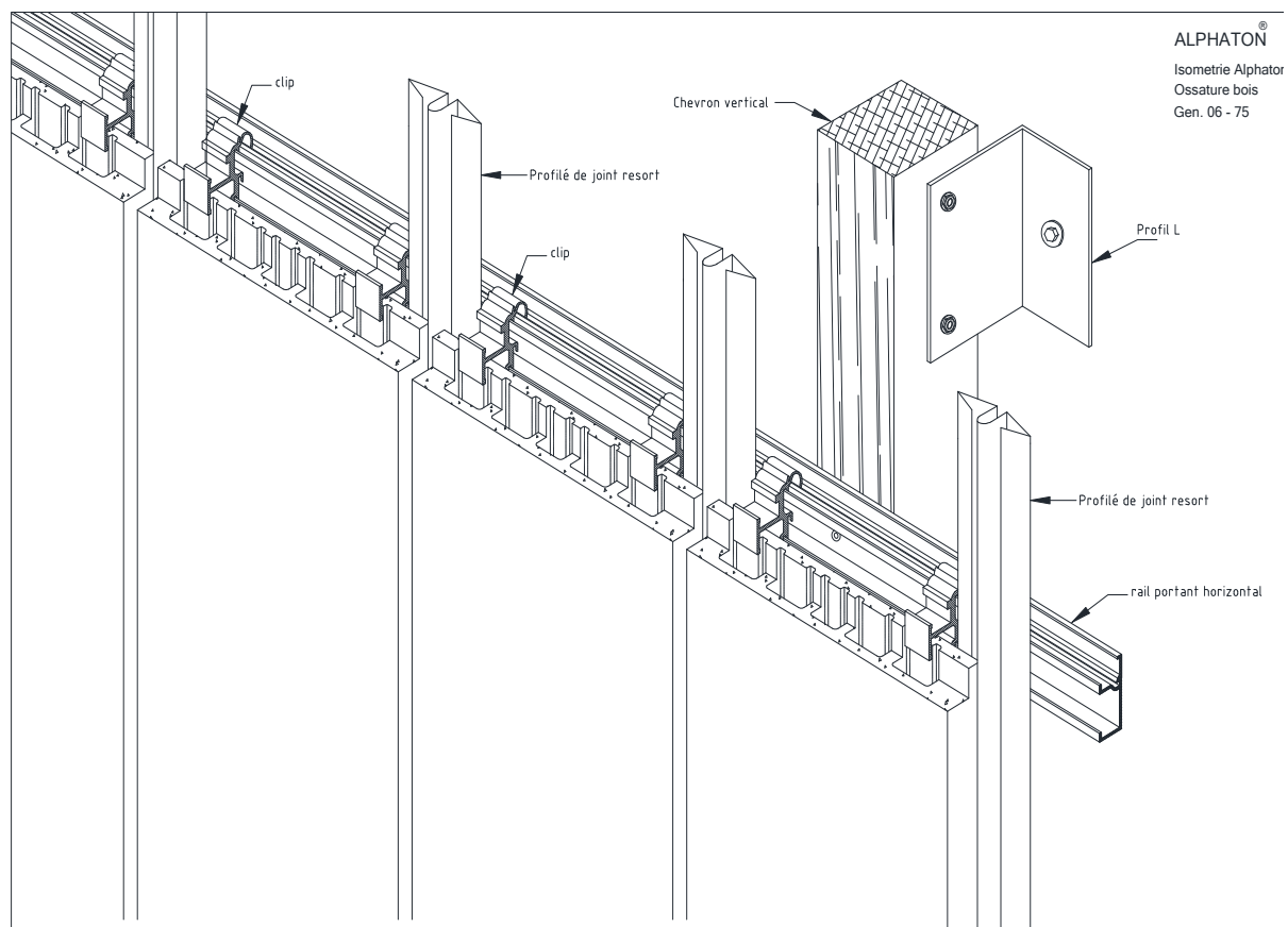
Figure 10 - Schéma de principe ossature bois - Vue isométrique - pose avec rail portant horizontal 06'75
