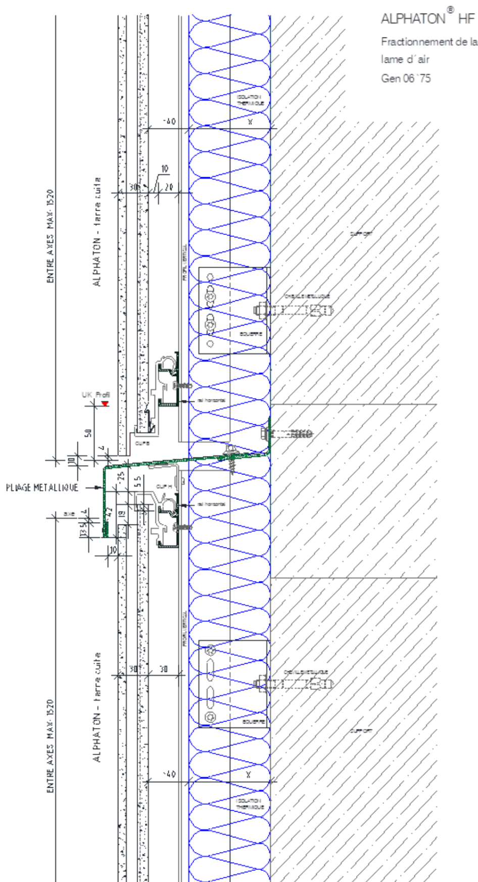
Figure 27 – Fractionnement de la lame d'air – bavette visible
