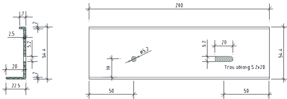
Figure 6bis - Pièce d'aboutage des rails horizontaux 06'75
