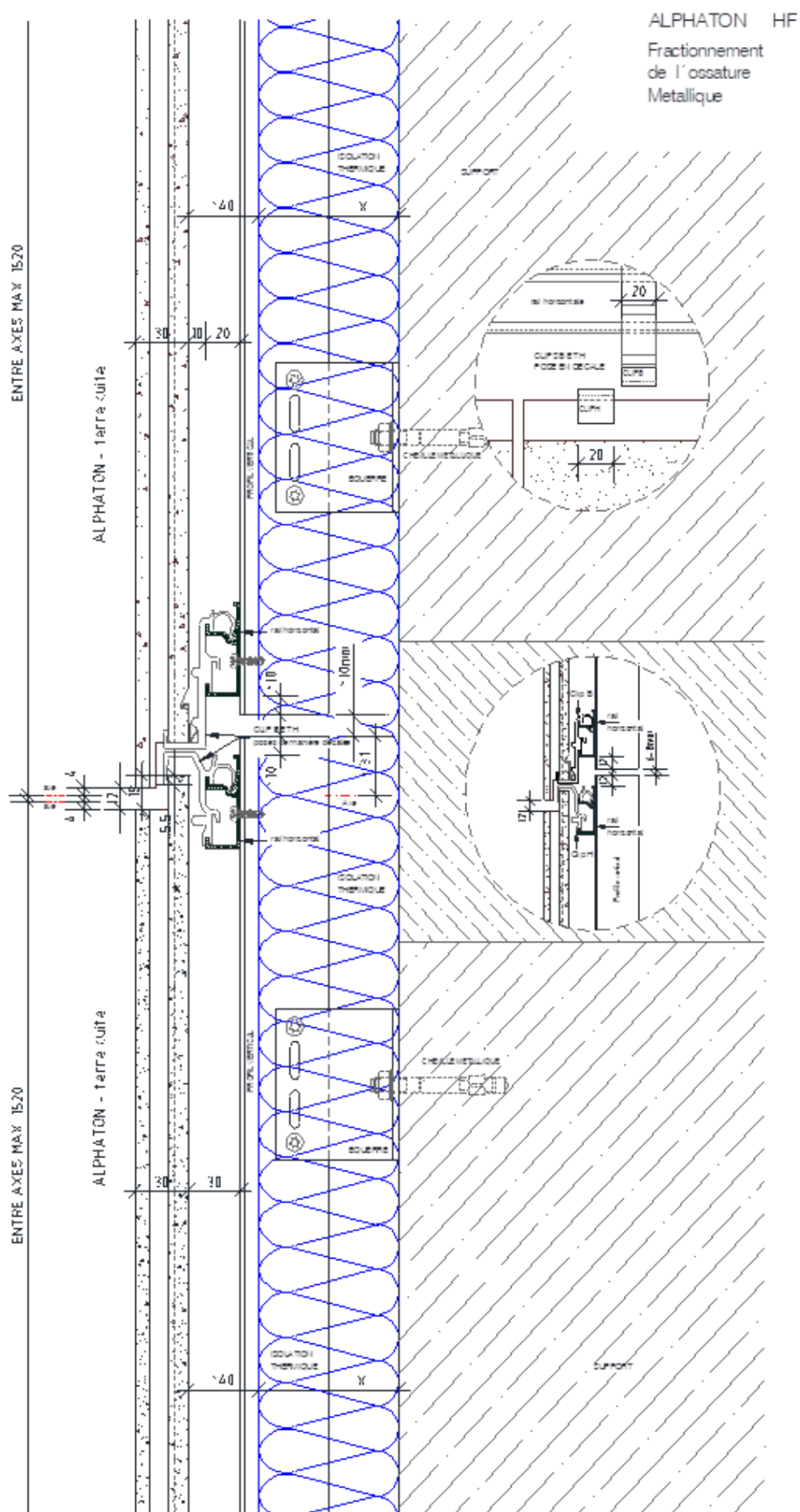
Figure 26 - Fractionnement de l'ossature aluminium bridée
