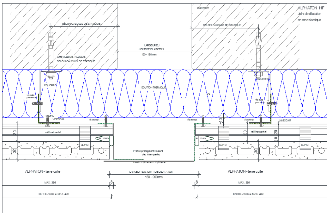
Figure B2 – Détail joint de dilatation de 12 à 15 cm
