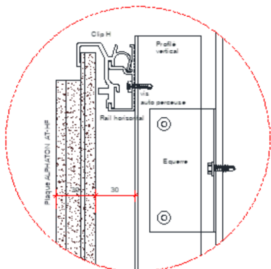
Coupe verticale - Clip haut
