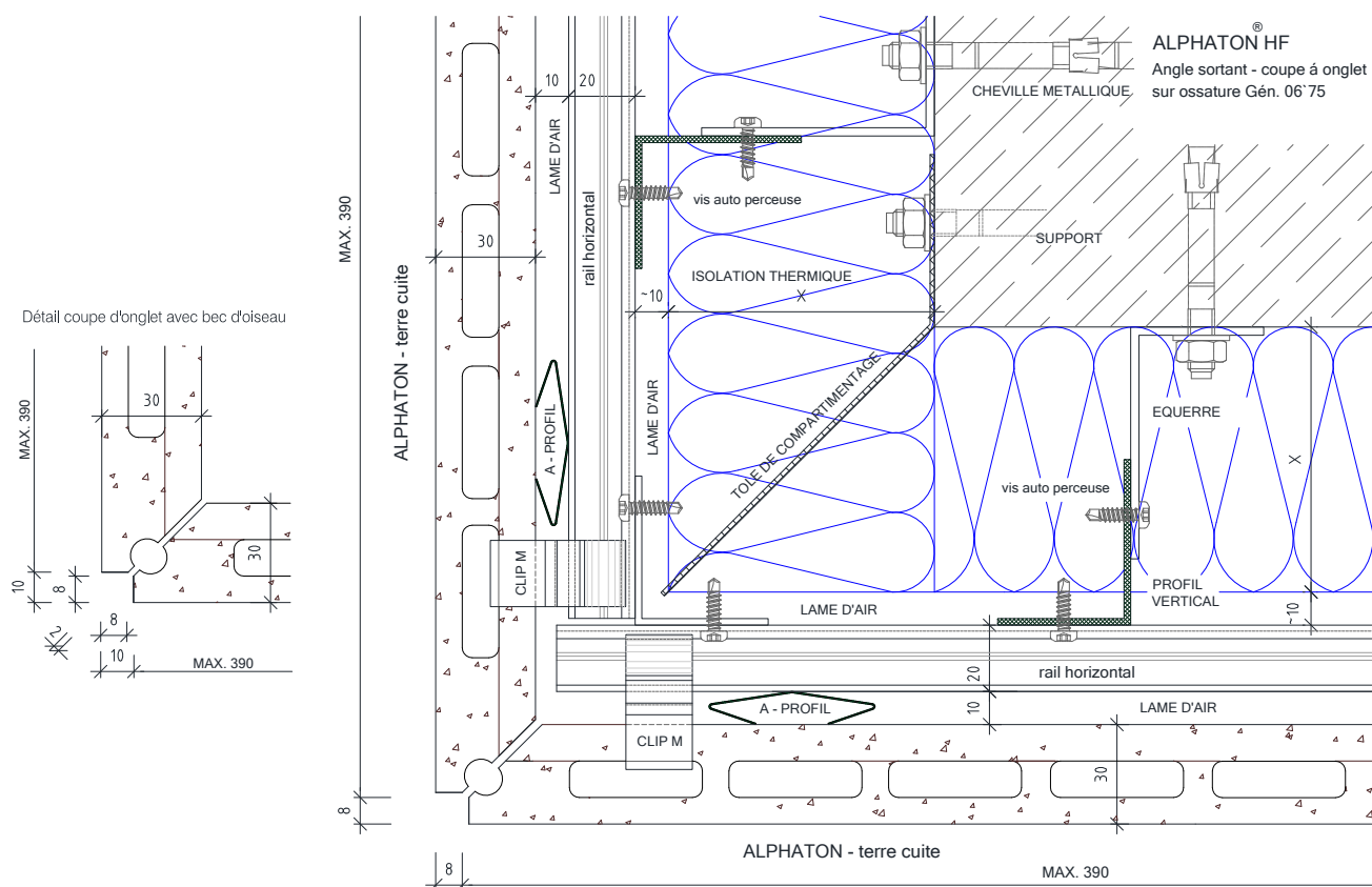
Figure 20 - Traitement des angles sortants - finition avec bardeaux à coupe d'onglet
