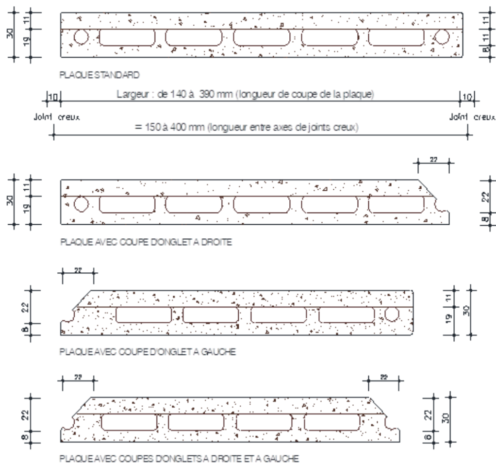
Figure 3 - Bardeaux d'angle et coupes d'onglet
