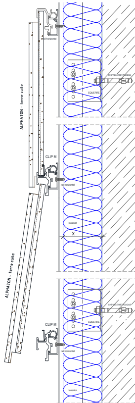
Figure 24bis - Montage des bardeaux – méthode 2
