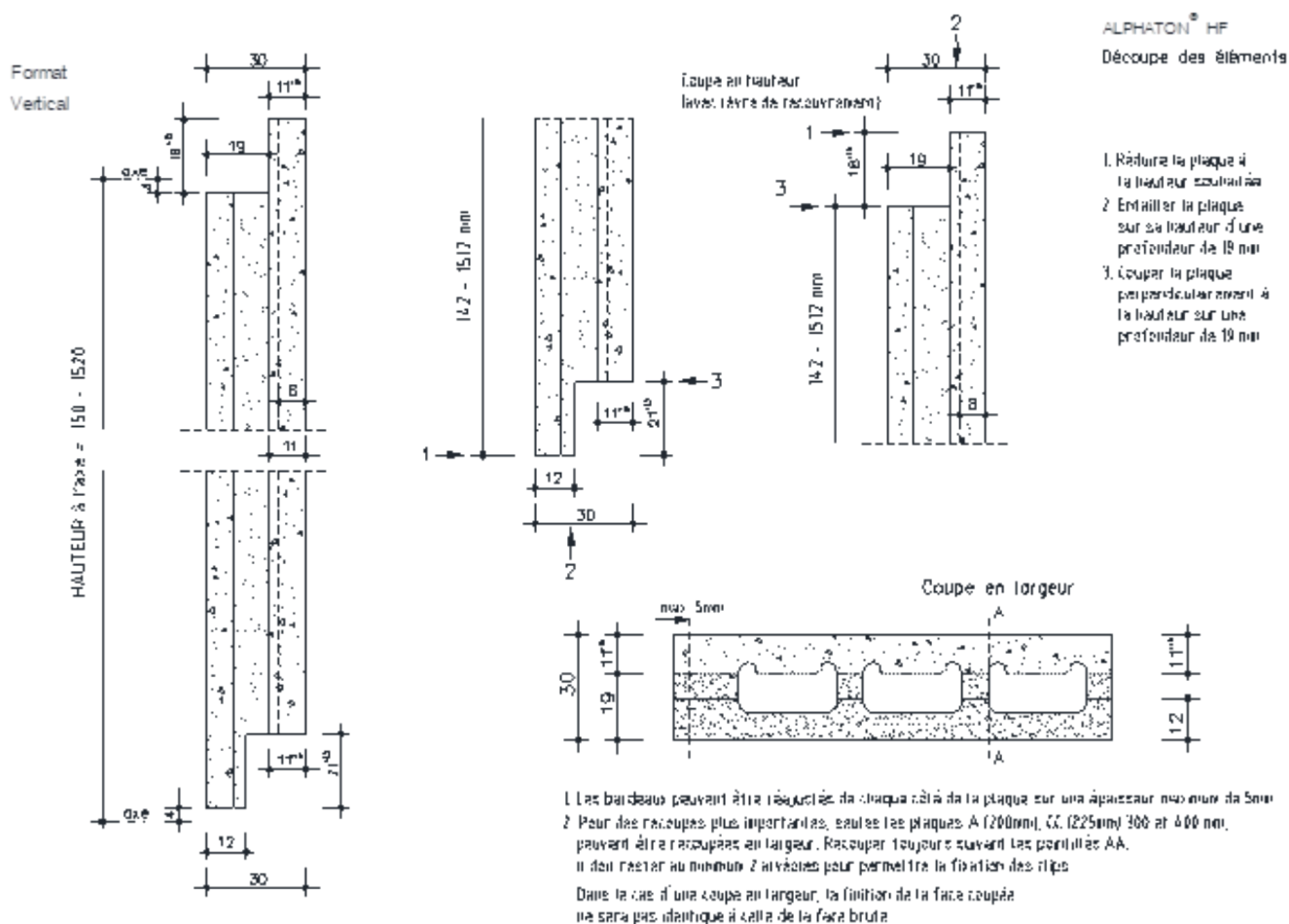
Figure 7 - Découpe des éléments terre cuite Alphaton® HF
