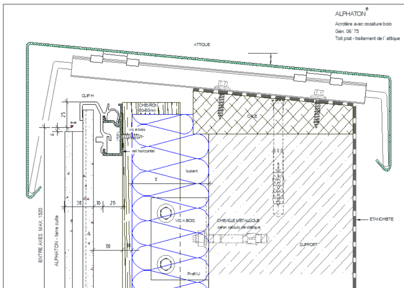
Figure 34 - Acrotère
