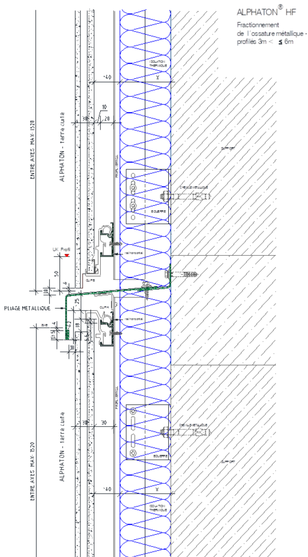
Figure 25bis - Fractionnement de l'ossature aluminium librement dilatable – montants de max. 6m
